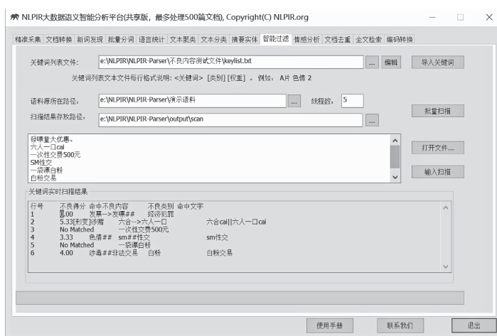
图 16 输入扫描
