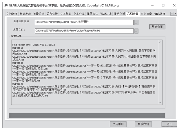
图 19 文档去重
