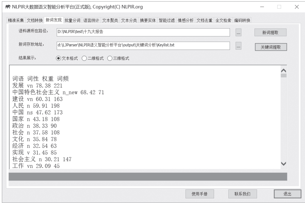
图 11 关键词提取
