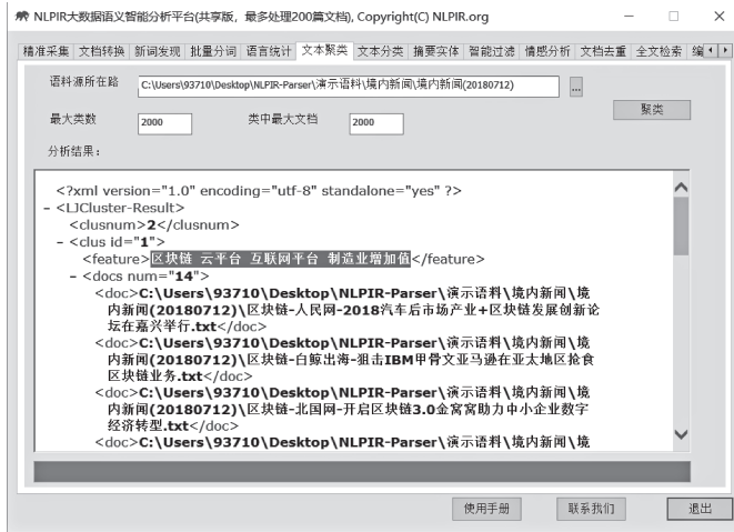
图 13 聚类
