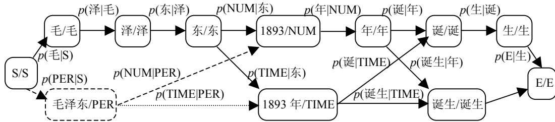
图 3.基于类的二元切分词图（原始字串为“毛泽东 1893 年诞生”）
