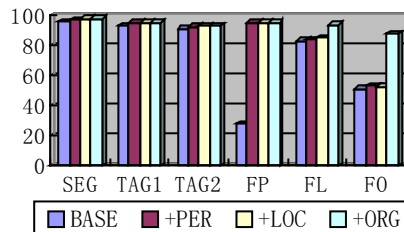
图 5.四种条件下的词法分析的性能指标
