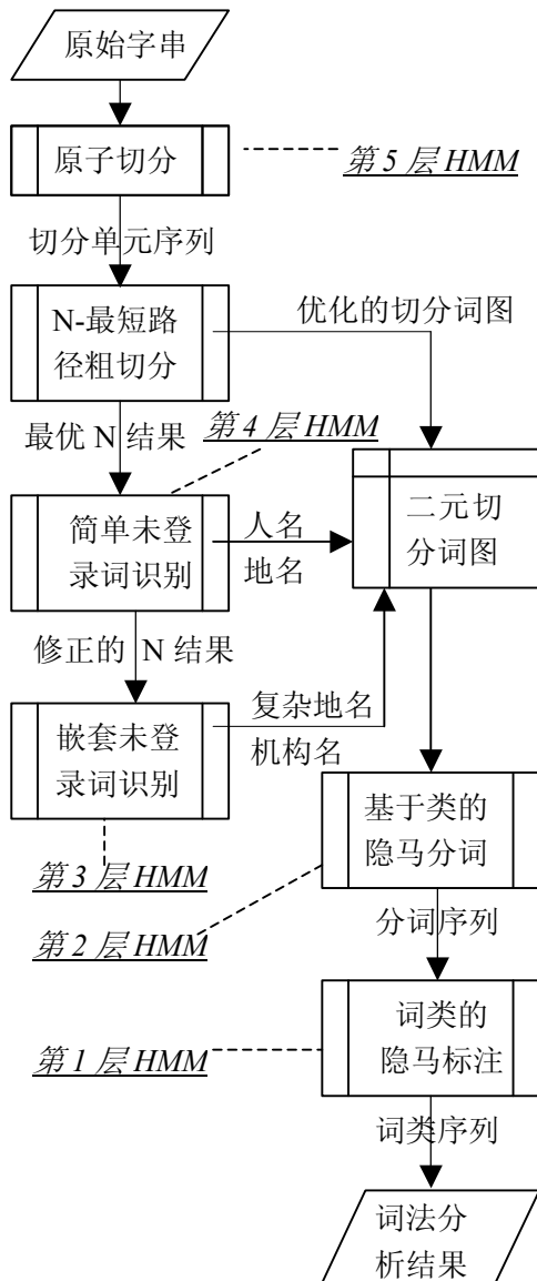
图 1. 基于 HHMM 的汉语词法分析框架
